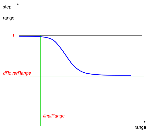
Fig. 7.1: Step limit.
